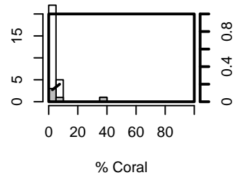
cupuladria.biporosa.b, bin :
