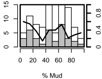
cupuladria.biporosa.b, bin :
