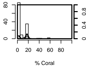
cupuladria.panamensis, bin
