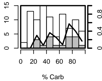
cupuladria.panamensis, bin
